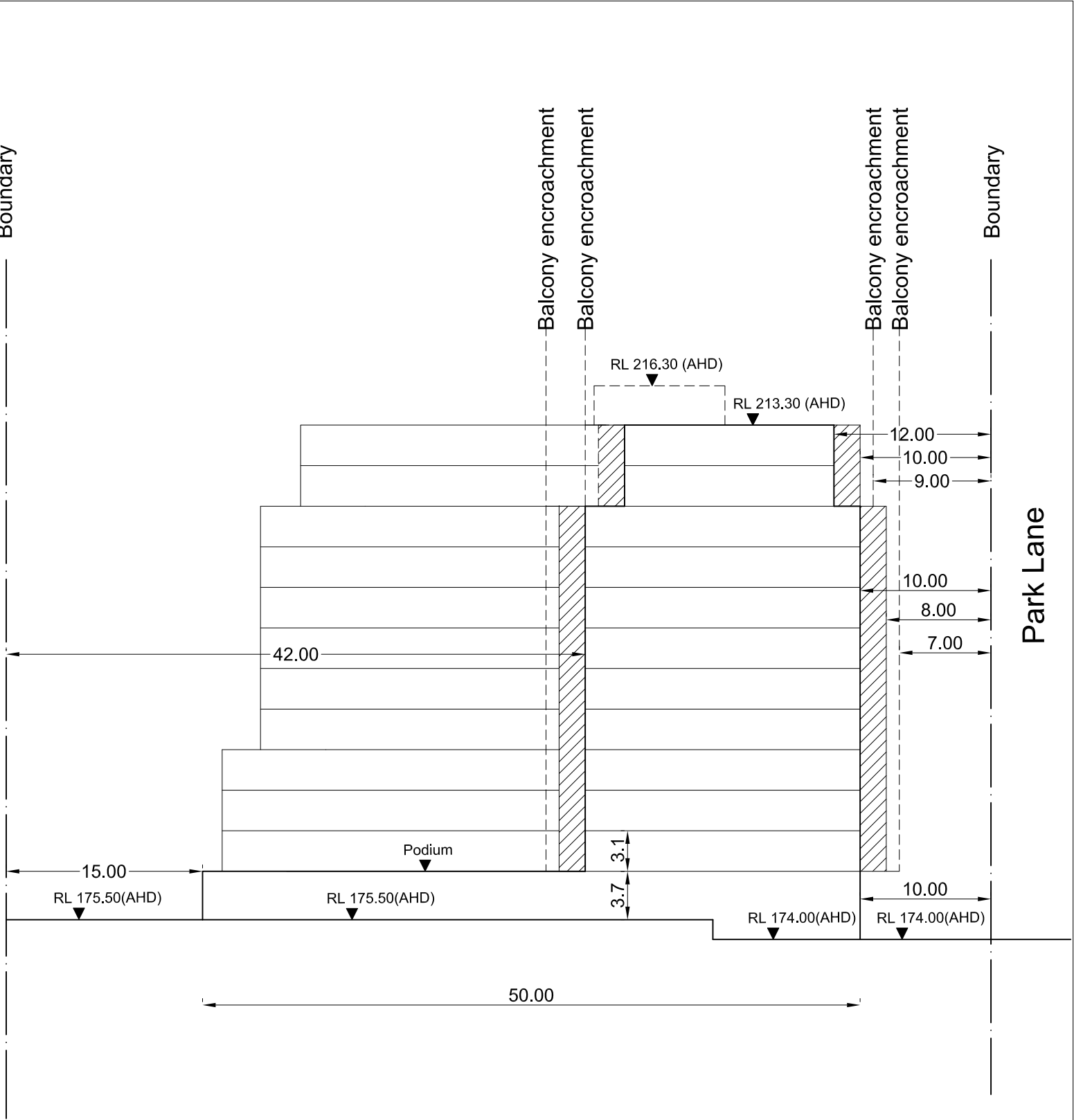
Section DD
